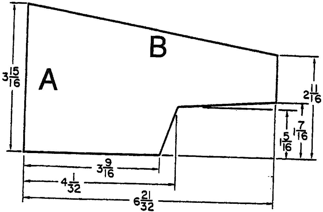
AILERON BELLCRANK TOOL
